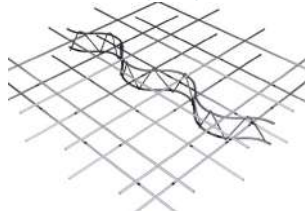
Distancier Zig Zag
