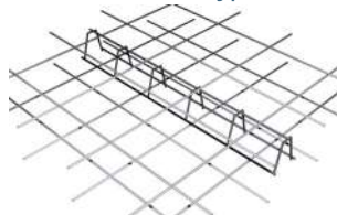
Distancier métal type A
