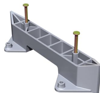
Talonnette avec clous
