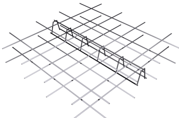
Distancier métal type A
