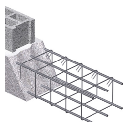
Semelles symétriques
